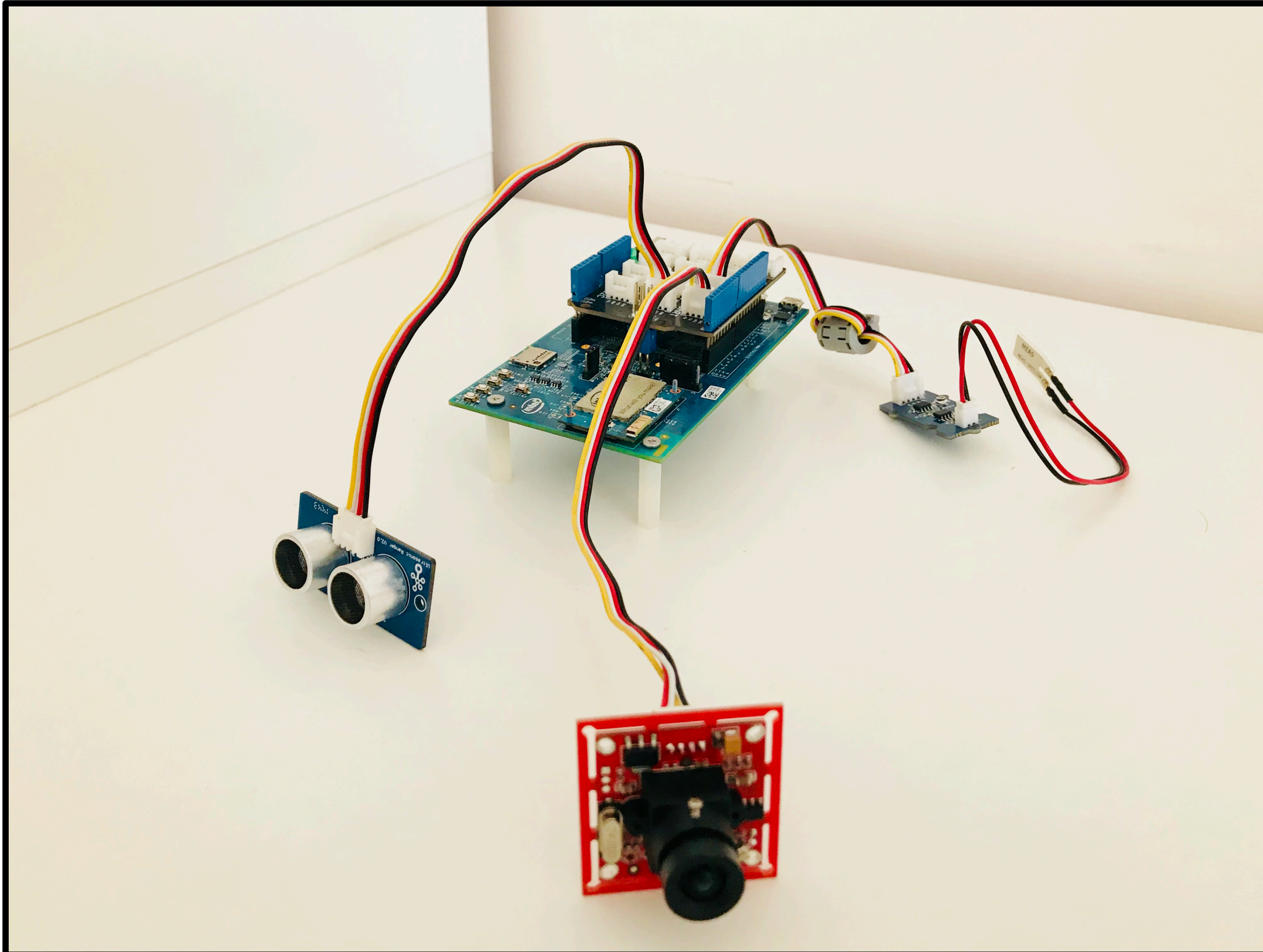
Prototipo HW/SW di portatarga connesso
